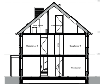
Doorsnede 1 : 100
