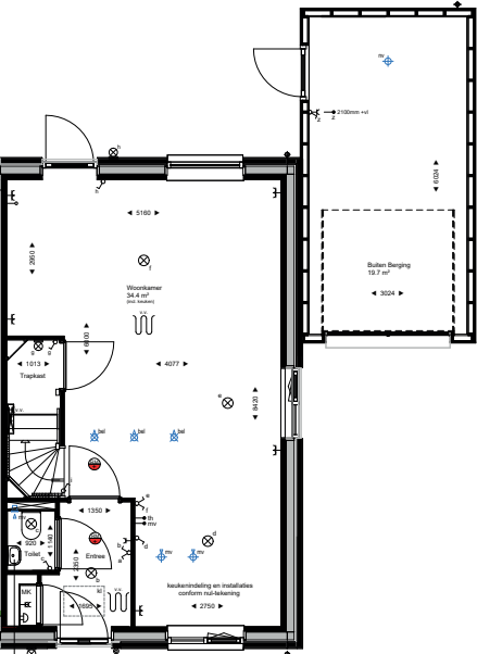
Begane grond 1 : 50
