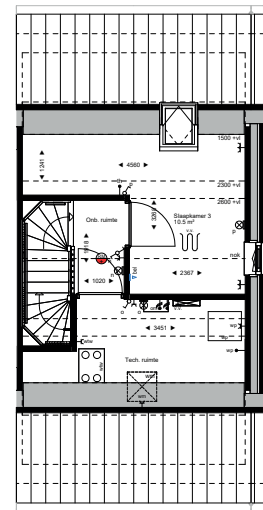
Tweede verdieping 1 : 50
