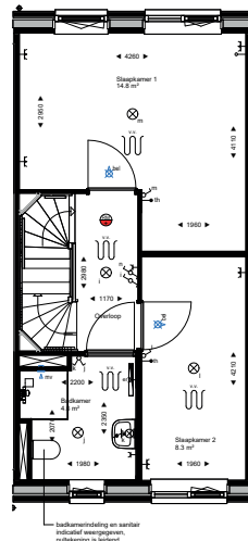
Eerste verdieping 1 : 50
