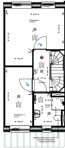
Eerste verdieping 1 : 50
