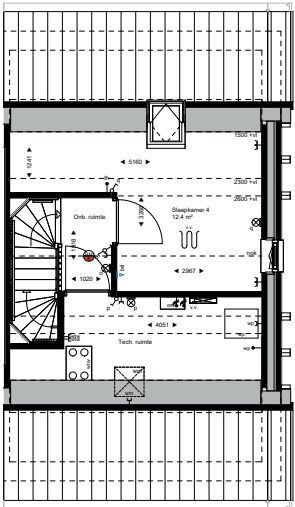
Tweede verdieping 1 : 50
