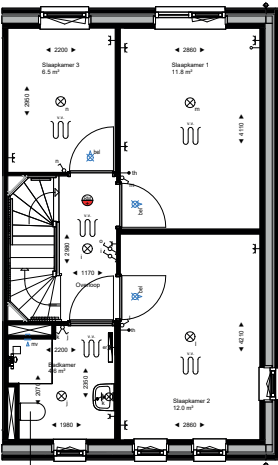
Eerste verdieping 1 : 50
