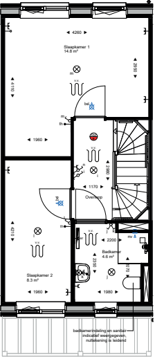
Eerste verdieping 1 : 50
