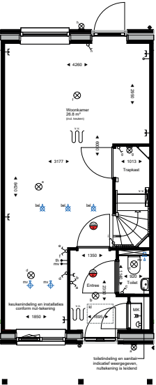
Begane grond 1 : 50
