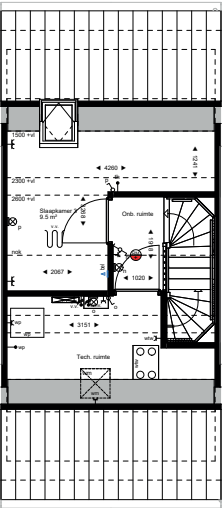
Tweede verdieping 1 : 50
