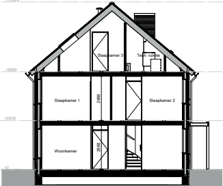
Doorsnede 1 : 100
