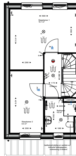
Eerste verdieping 1 : 50
