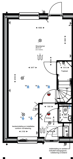
Begane grond 1 : 50
