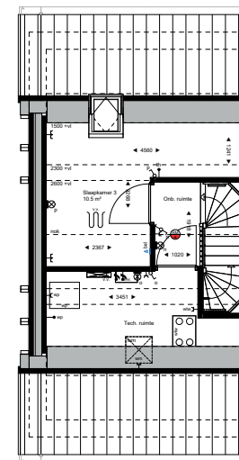
Tweede verdieping 1 : 50
