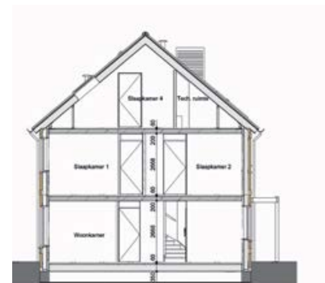
Doorsnede
