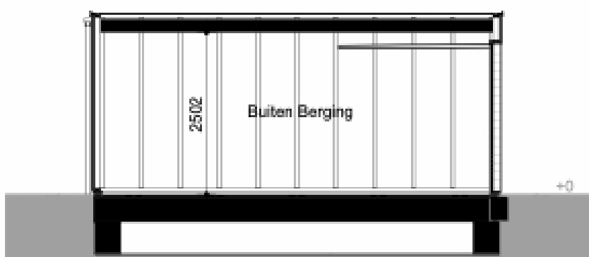
Doorsnede 1 : 100
