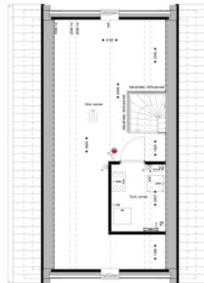
Tweede verdieping 1 : 50
