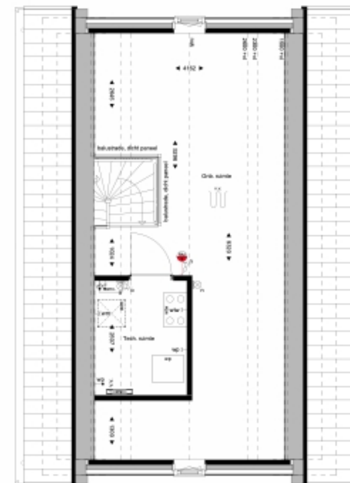
Tweede verdieping 1 : 50
