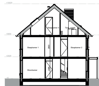
Doorsnede 1 : 100
