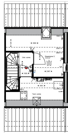
Tweede verdieping 1 : 50
