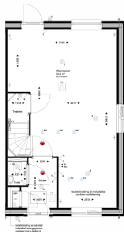
Begane grond 1 : 50
