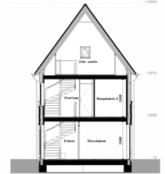
Doorsnede 1 : 100
