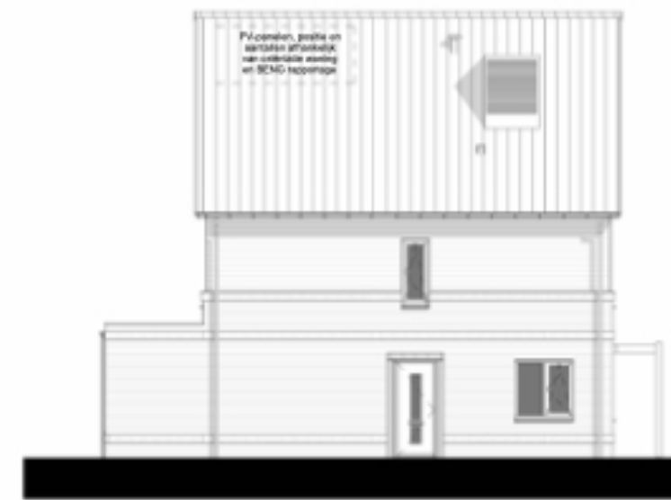
Linker zijgevel 1 : 100
