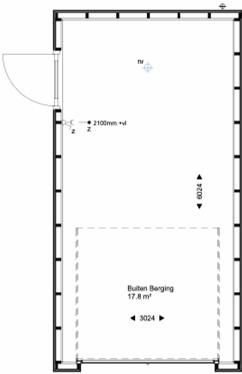
Begane grond 1 : 50
