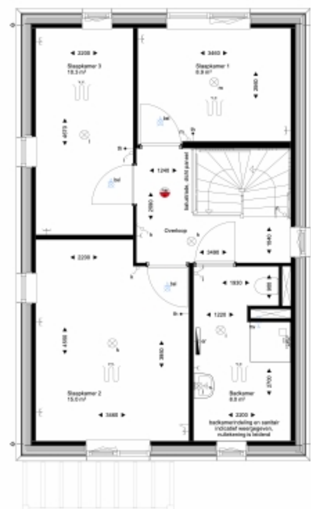
Eerste verdieping 1 : 50
